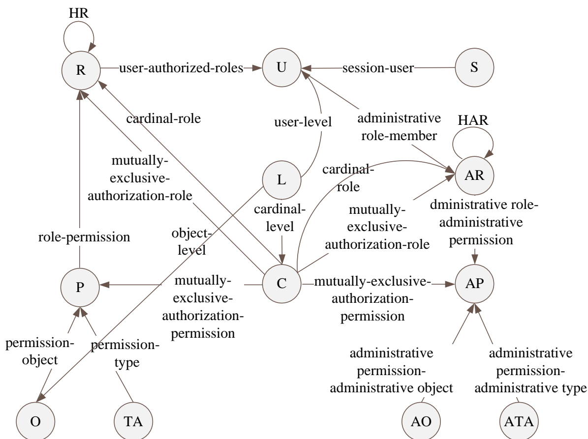
Рис. 1. Обобщенная модель разграничения прав доступа
