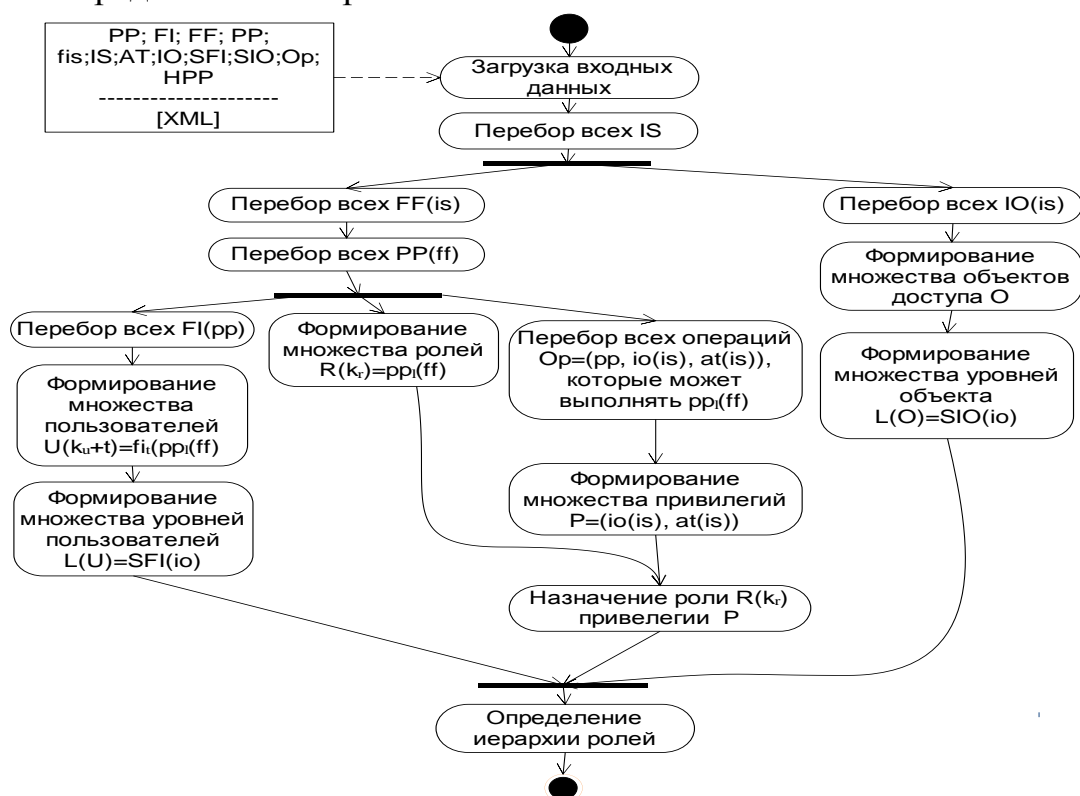
Рис. 6. Детализация блока «Выгрузка данных из модели бизнес-процесса»
