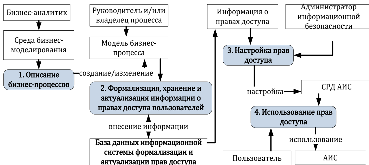
Рис. 2. Потоки данных в информационной системе формализации и актуализации прав доступа
