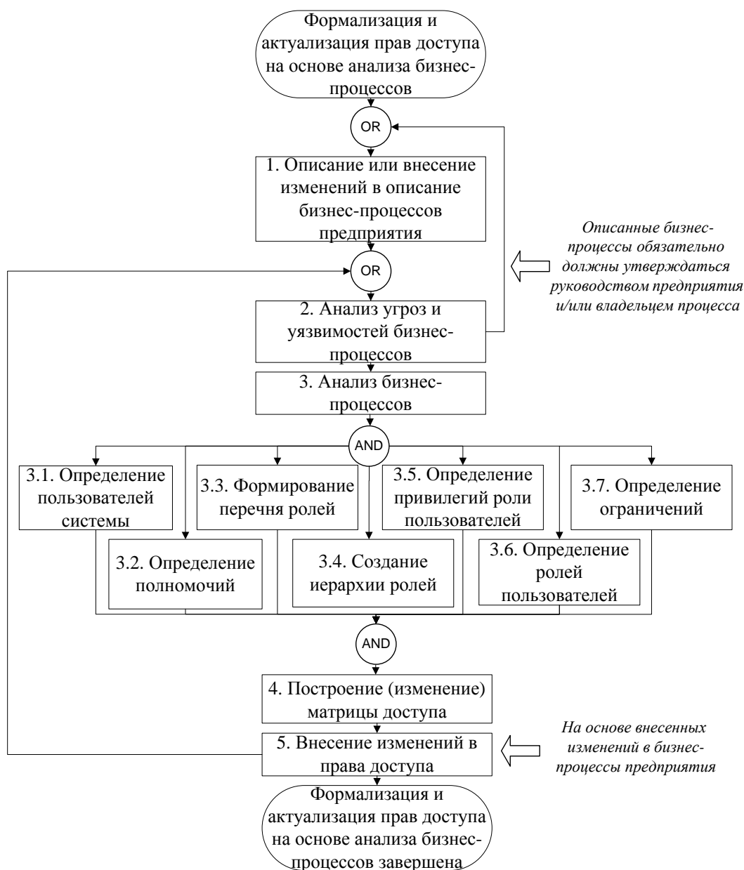
Рис. 3. Этапы формализации и актуализации прав доступа на основе анализа бизнес-процессов предприятия
